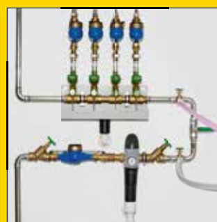
Preplachovanie rozvodov pitnej vody (S/SL/SLW)
