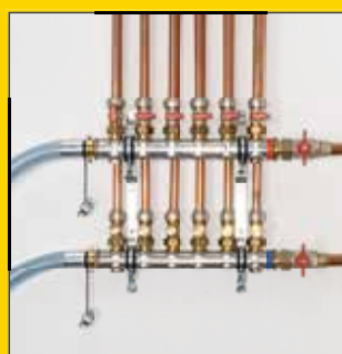
Preplachovanie radiátorov a plošných vykurovacích systémov (S/SL/SLW)
